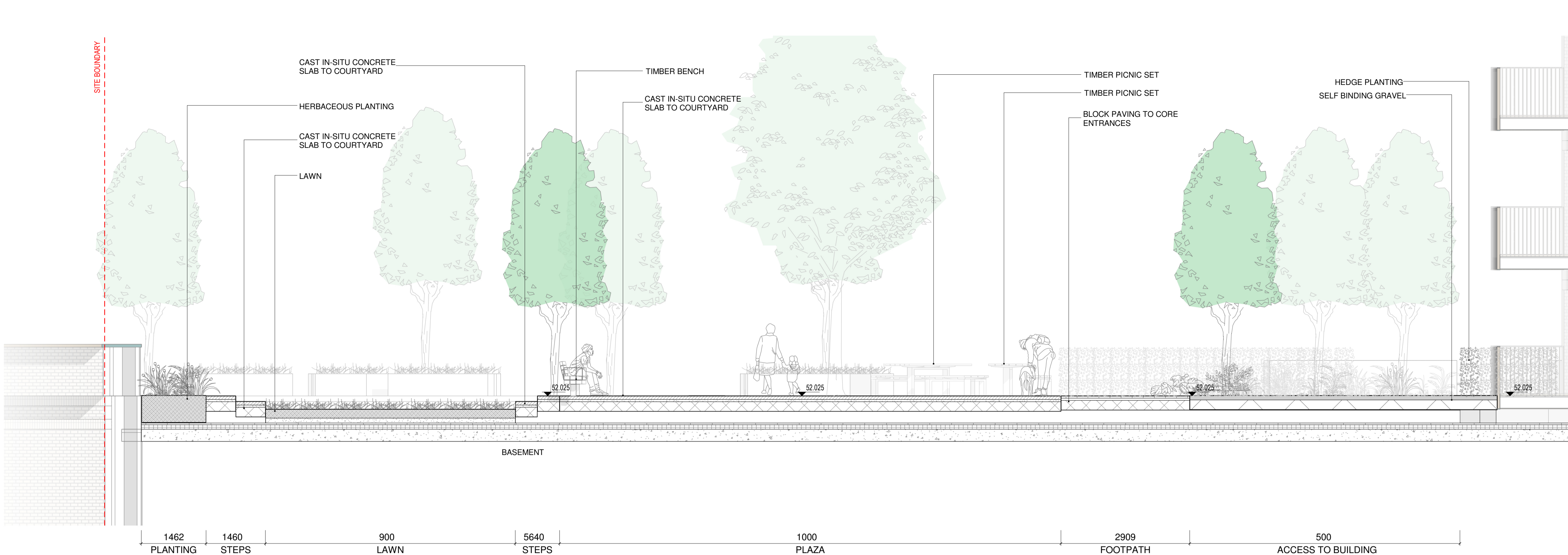
7 SECTION 07 SCALE: 1 : 50 @A1
