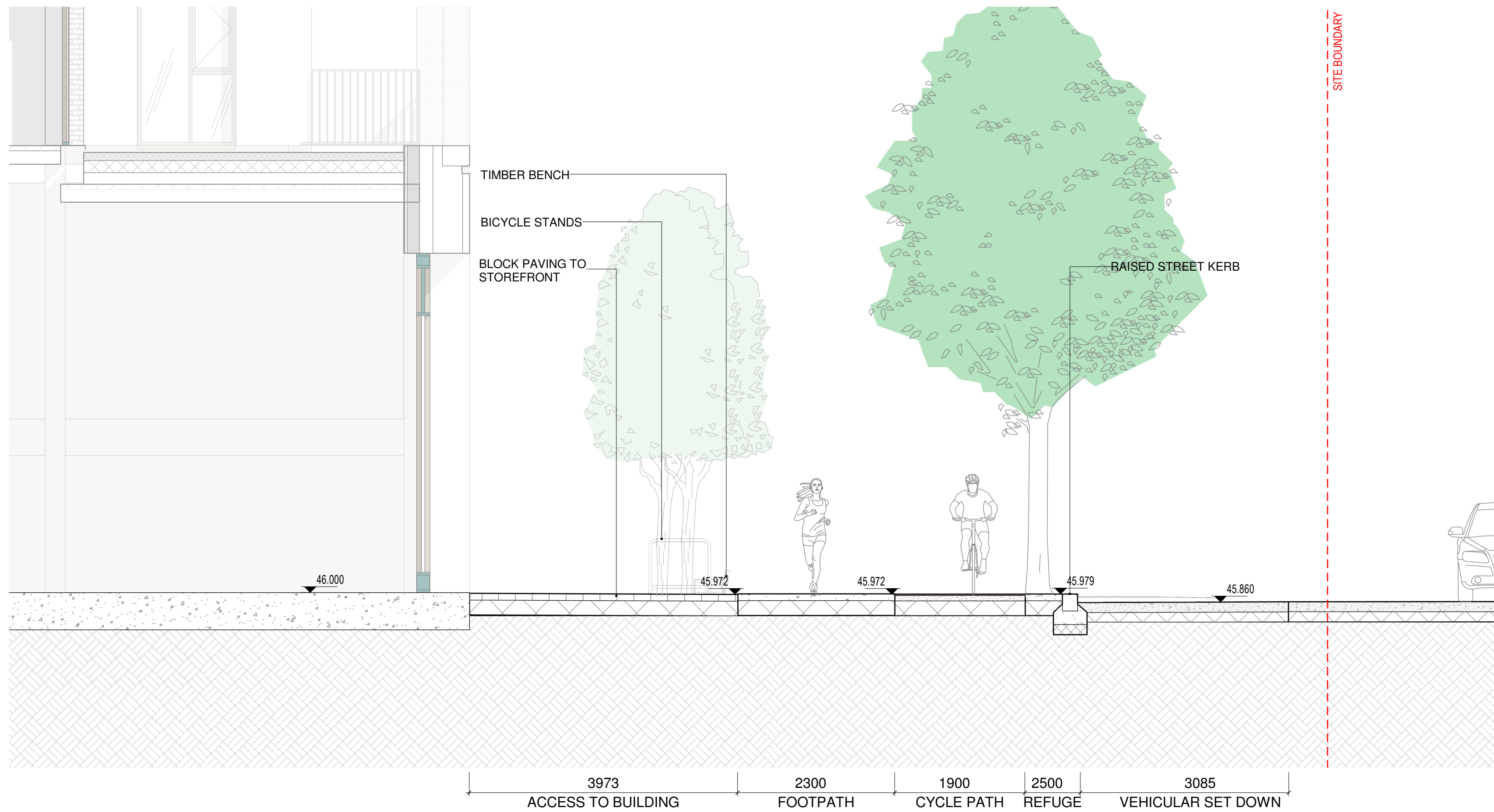
3 SECTION 03 SCALE: 1 : 50 @A1
