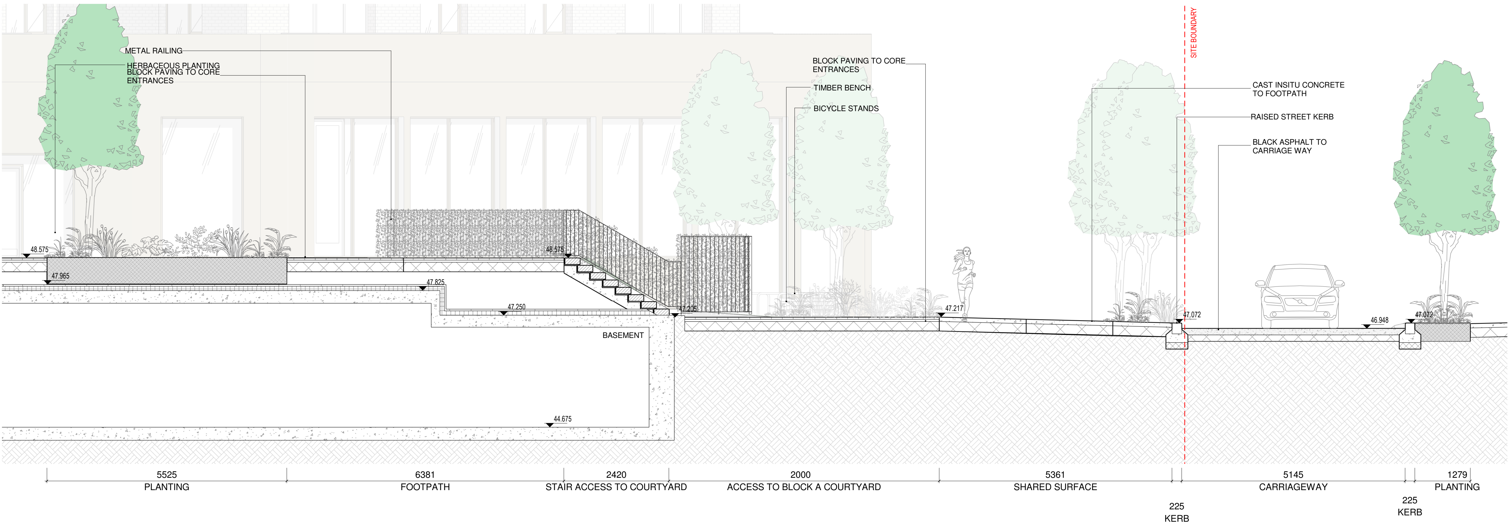
4 SECTION 04 SCALE: 1 : 50 @A1
