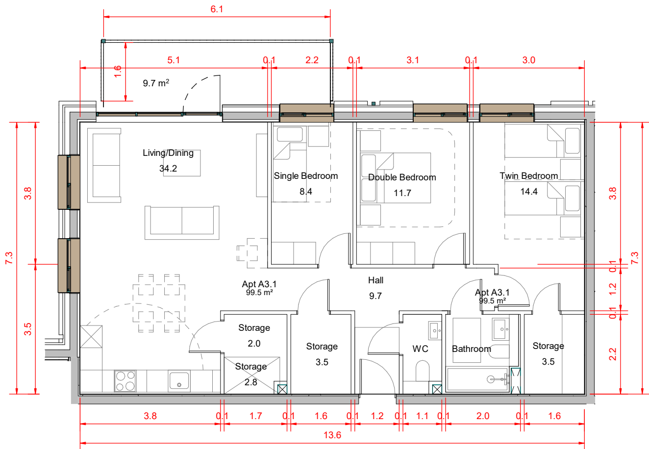
Apt A3.1 1 : 100
