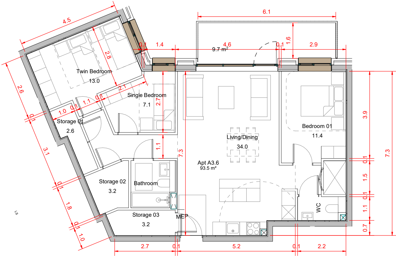
Apt A3.6 1 : 100
